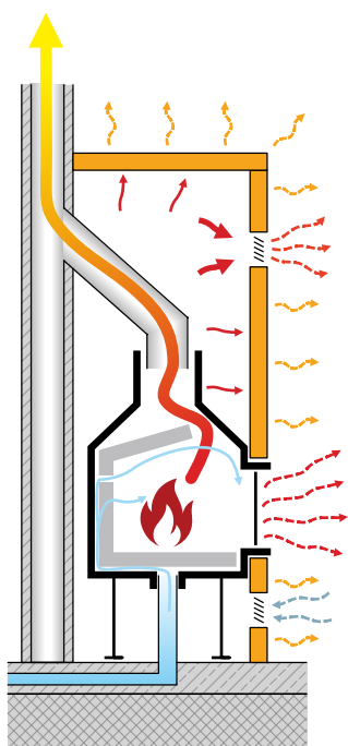
Toplozračno akumulacijski kamin - odprte rešetke
