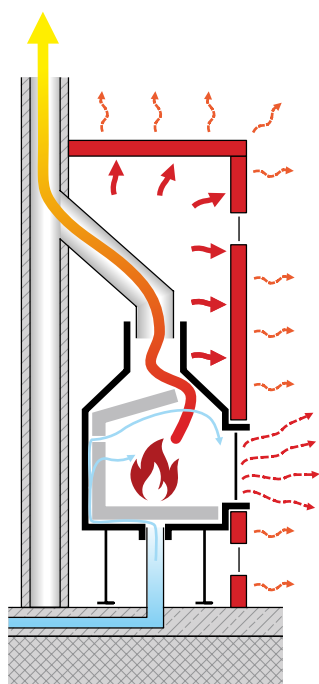
Toplozračno akumulacijski kamin - zaprte rešetke
