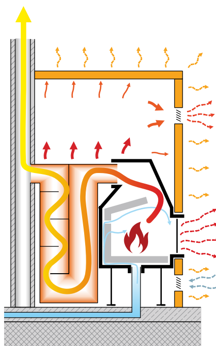
Akumulacijska peč - z dimovodnim sistemom
